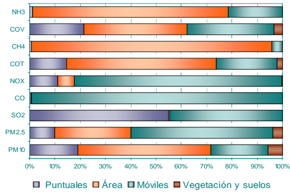
Gráfica 15. Contribución de emisiones por tipo de fuente, 2004
